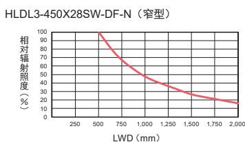
※1 光轴上的辐射照度 ※2 光源与被测物体之间的照射距离 相对辐射照度图表 (LWD 特性)
